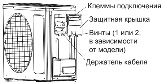
Клеммы подключения проводов
