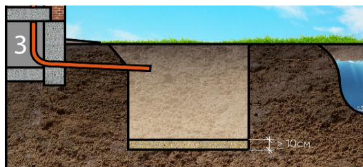
Устройство песчаной подушки. Минимум 10 см.
