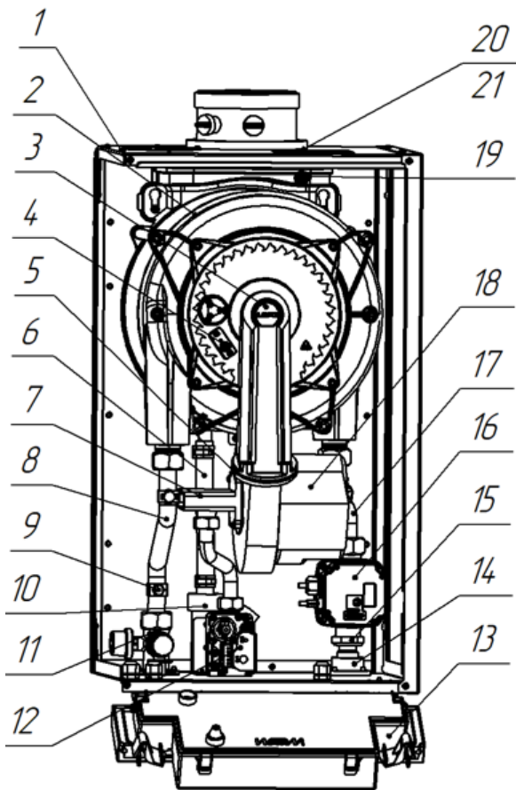
Рис. 10.2. Общая схема и основные элементы котла 49 кВт / 60 кВт
