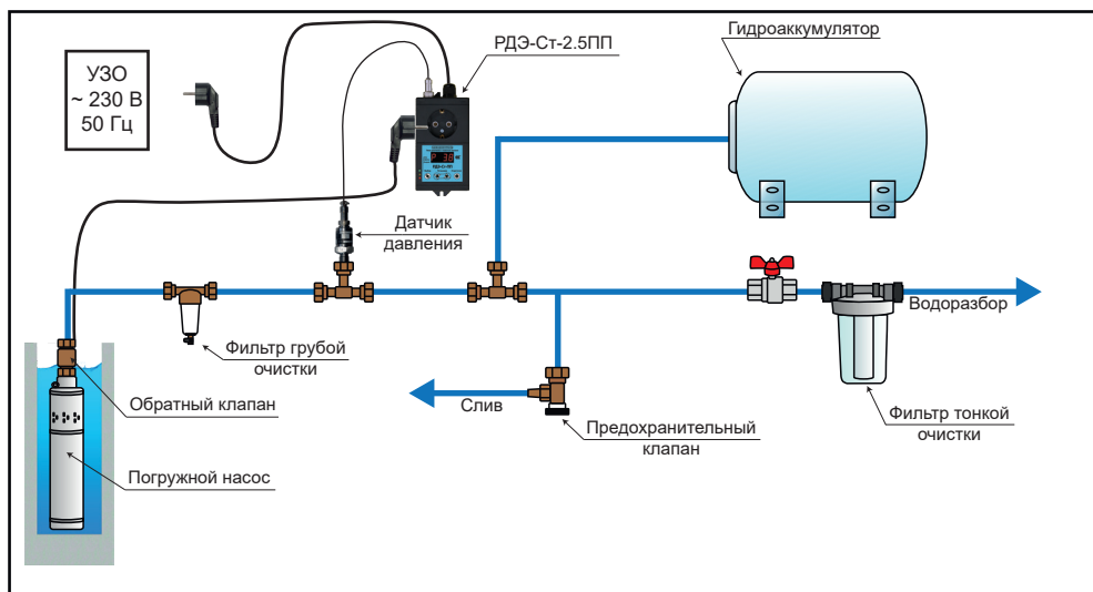
Пример 4. Подключение РДЭ-Ст-2.5-ПП к погружному насосу.
