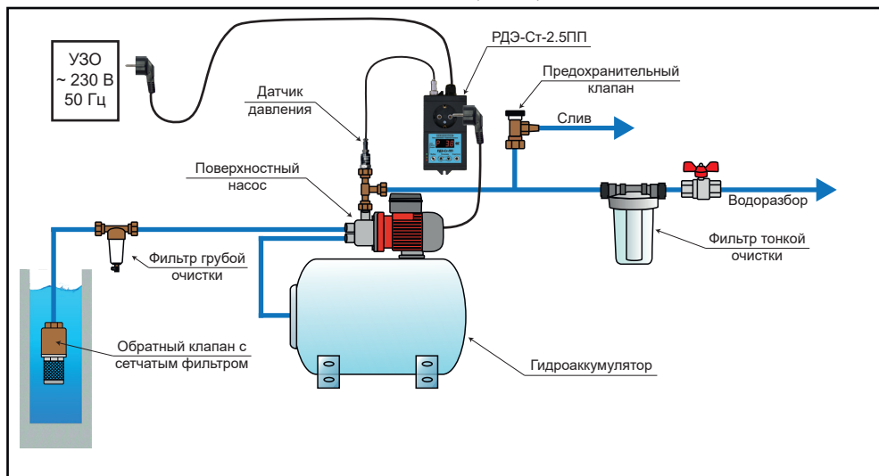
Пример 3. Подключение РДЭ-Ст-2.5-ПП к поверхностному насосу или насосной станции.
