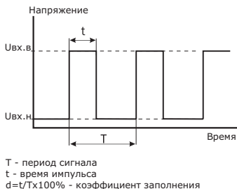
Рис. 16 Характеристики ШИМ-сигнала
