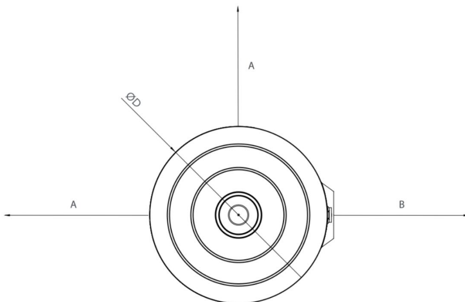
Рис. 1 Монтажные расстояния
