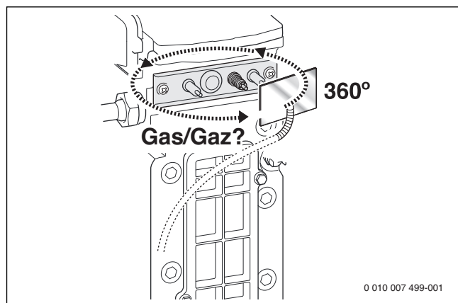
Рис. 56 Проверка герметичности
