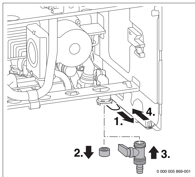
Рис. 25 Установка крана для заполнения и слива
