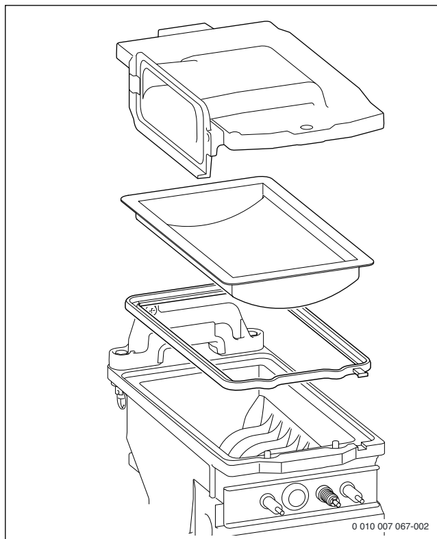
Рис. 58 Горелка
