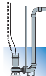
Установка с донным соединительным устройством
