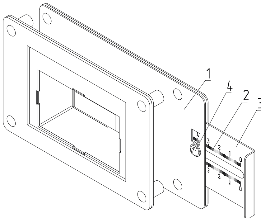
Рис.16 Заслонка вентилятора
