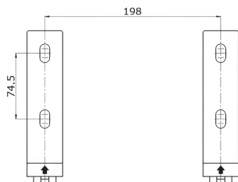
Рис. 8 Монтажные габариты комплекта настенного монтажа
