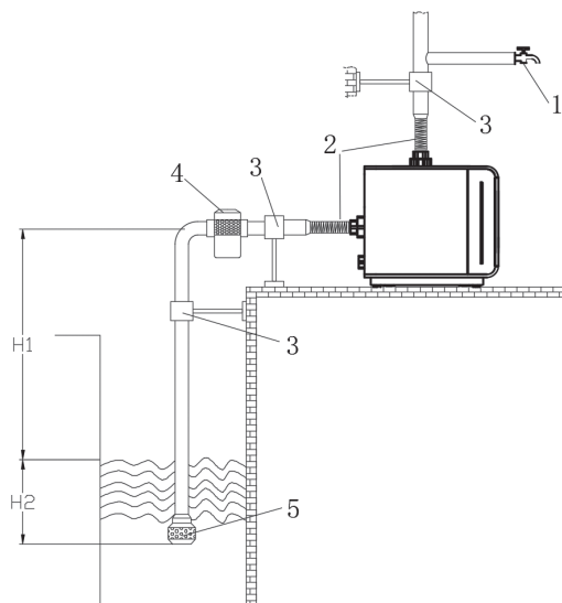
Рис. 12 Подача воды из колодца/скважины
