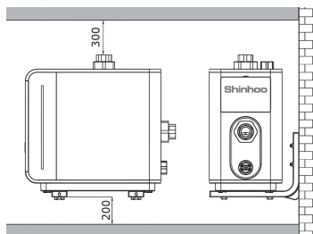
Рис. 7 Требуемое пространство при установке комплекта настенного монтажа
