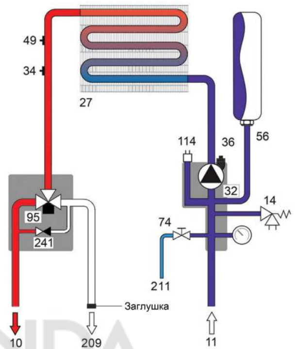
Рис. 18. Отопительный контур
