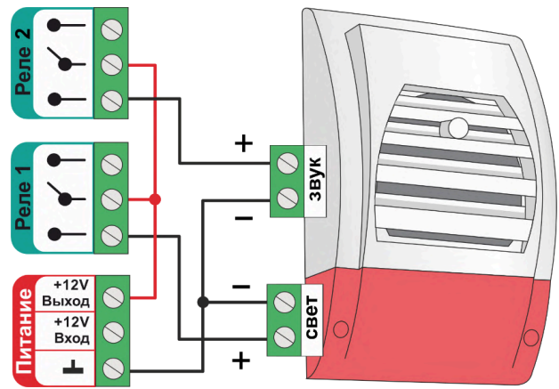
Схема подключения свето-звукового оповещателя к релейному выходу
