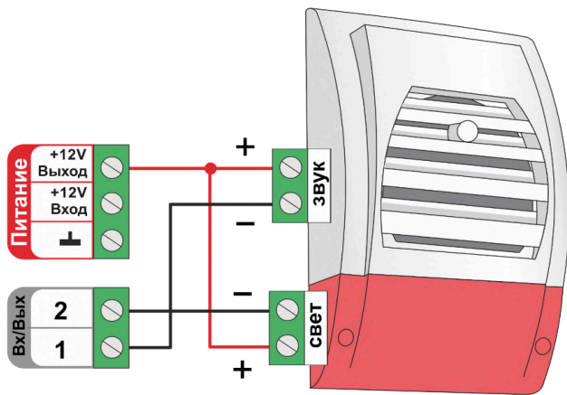
Схема подключения свето-звукового оповещателя к выходу ОК
