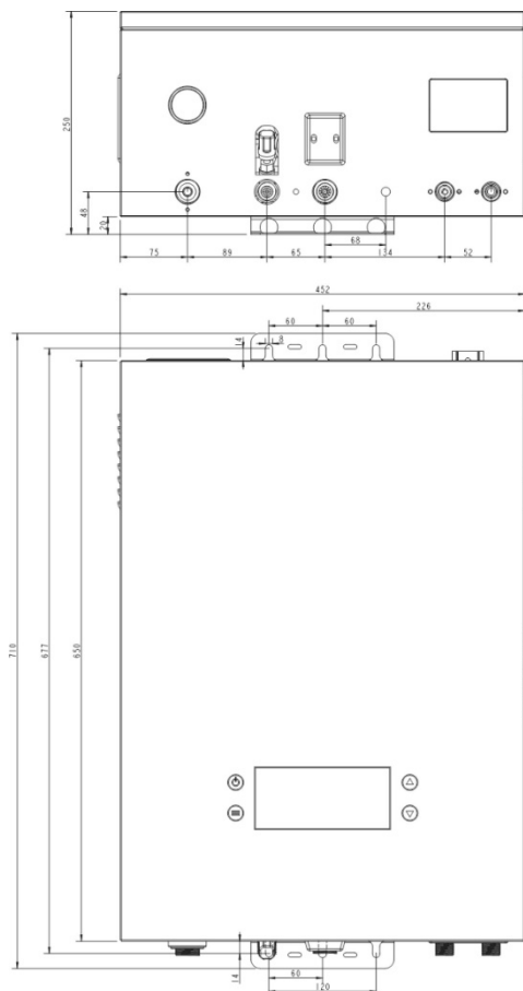
Рис.2. Габаритные размеры
