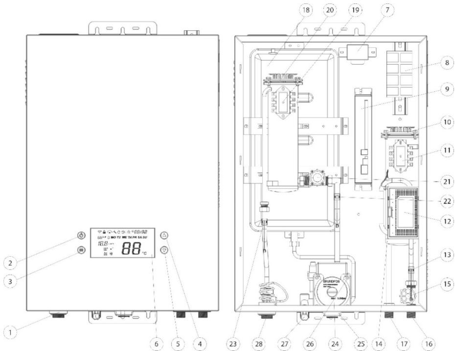
Рис. 1. Конструкция изделия
