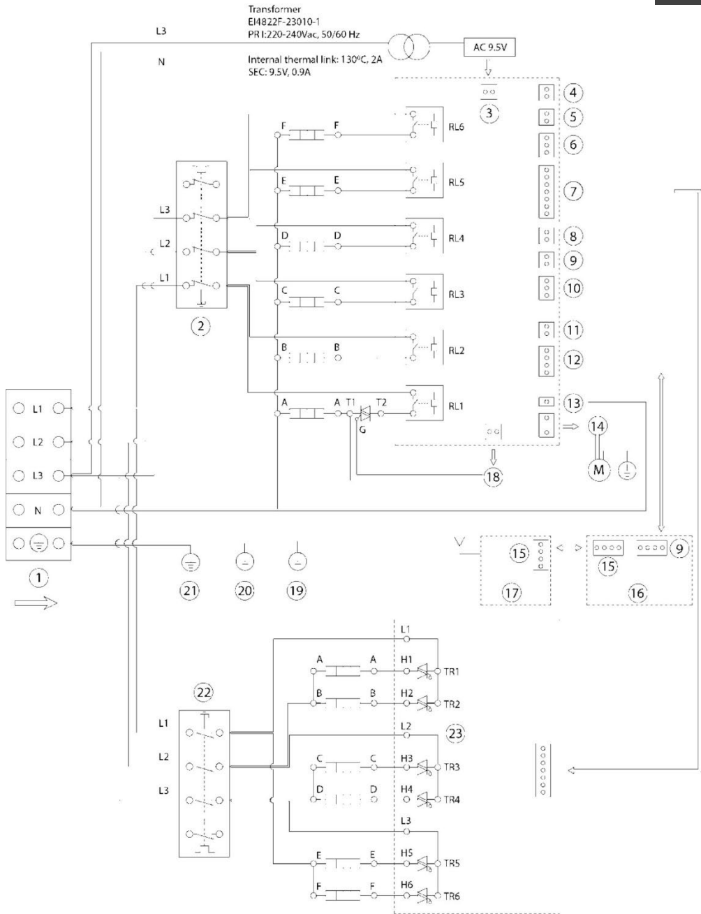
Рис.11. Электрическая схема
