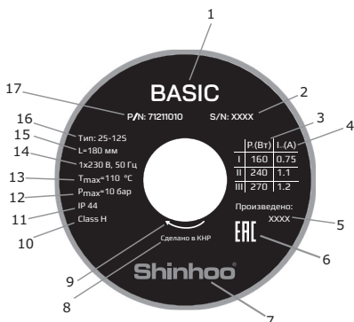
Рис. 2 Пример фирменной таблички
