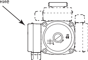
Рис. 6 Возможное положение клеммной коробки
