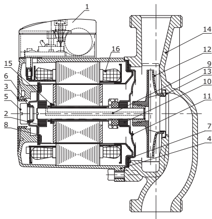
Рис. 1 Разрез насоса BASIC, BASIC S
