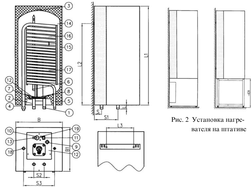
Рис. 1 Конструкция нагревателя
