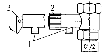
Рис. 4 Предохранительный клапан 1. водосливное отверстие предохранительного клапана, 2. головка, 3. рычаг
