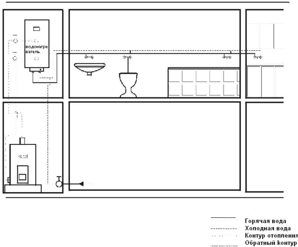
Рис. 1 ВОДОНАГРЕВАТЕЛЬ НАКОПИТЕЛЬНЫЙ КОМБИНИРОВАННЫЙ РАСПРЕДЕЛЕНИЕ ГОРЯЧЕЙ ВОДЫ
