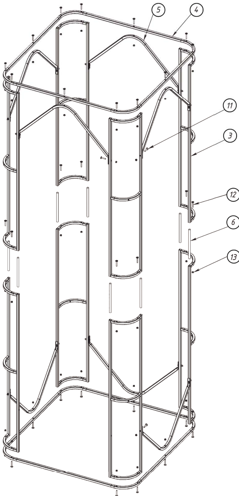
Рис. 1. Сборка каркаса.
