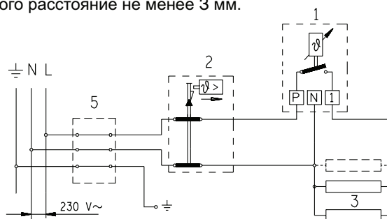
Электрическая схема
