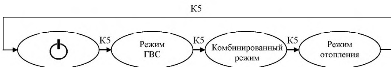
Рис. 5. Последовательность смены режимов работы котла
