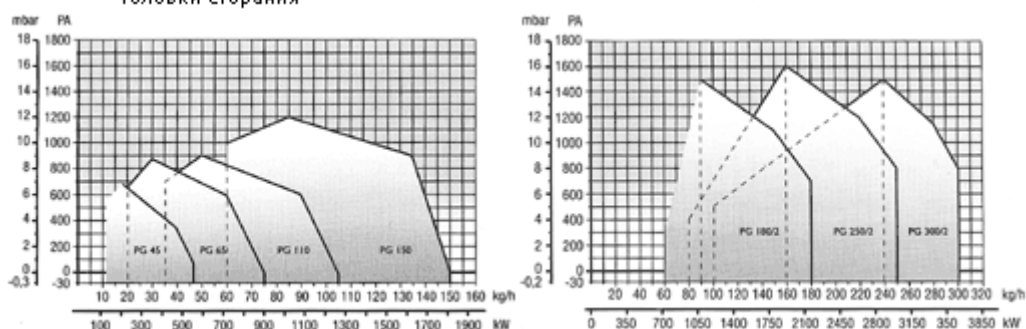
мощность в кВт в зависимости от противодавления в камере сгорания
