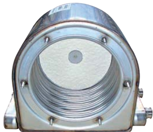
б) Первичный теплообменник в конденсационных котлах
