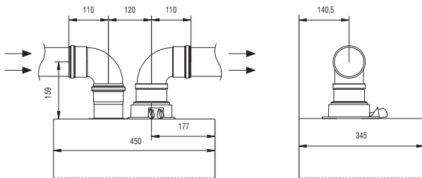
NUVOLA Duo-tec
