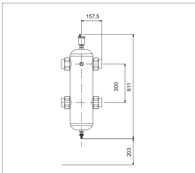
Гидравлический разделитель 2"
