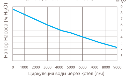
Характеристика расход - напор насоса из гидравлического комплекта POWER HT 45-150 кВт
