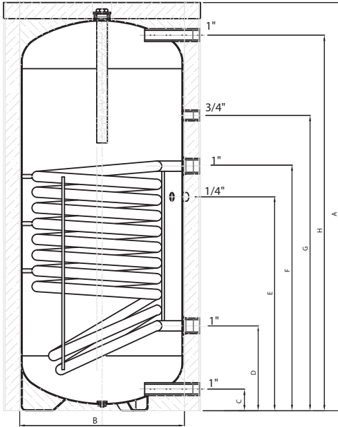
UB 300-400 SC
