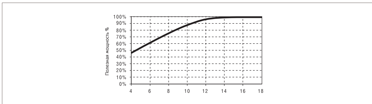
График зависимости полезной мощности от входного давления для котла ECO Four 240F
