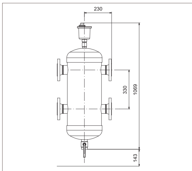
Гидравлический разделитель DN65
