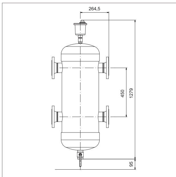
Гидравлический разделитель DN100
