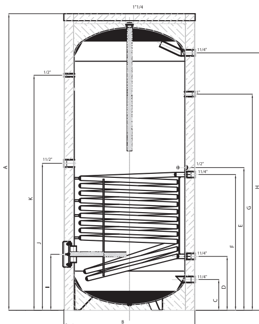
UB 1000-2000 SC
