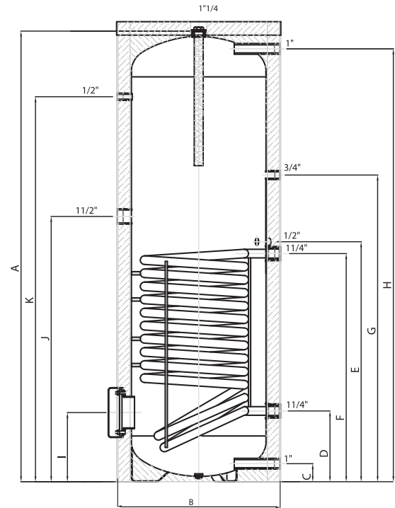
UB 200 SC
