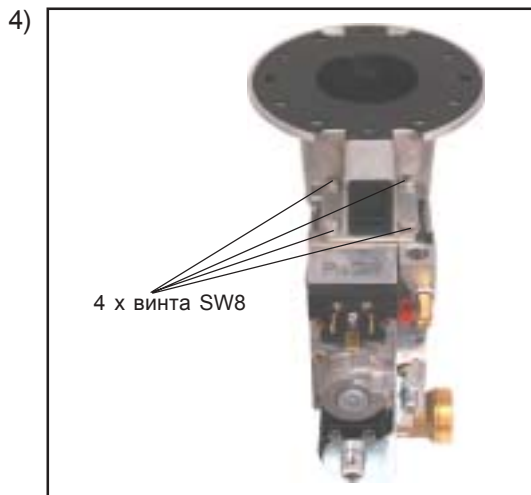
Отсоединить комбинированный газовый клапан от смешивательной камеры (отвинтить 4 винта SW8).
