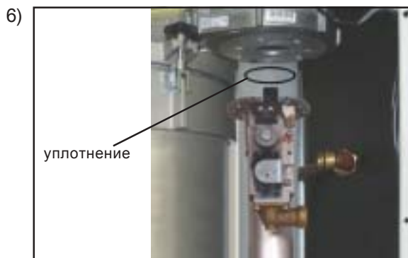
При обратной сборке газовой дроссельной шайбы, газового комбинированного клапана и воздухозаборного патрубка, вложить смазанное силиконом уплотнение в соответствующий паз вентилятора и смонтировать смешивательную камеру.
