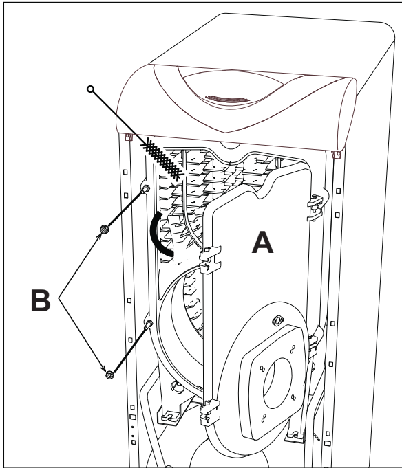
рис. 3 - Очистка котла
