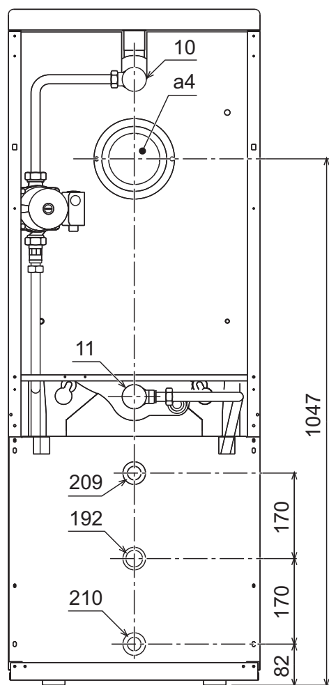
рис. 6 - Вид сзади
