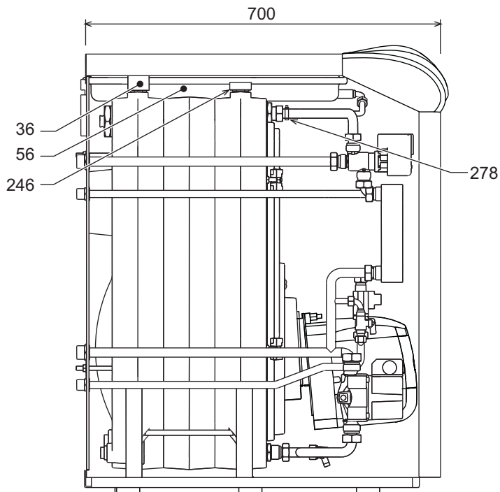
рис. 19 - Вид сбоку
