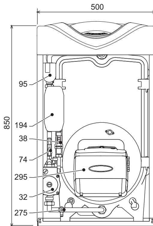
рис. 18 - Вид спереди
