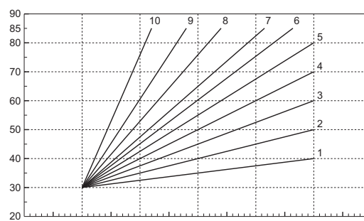
рис. 13 - Компенсационные характеристики
