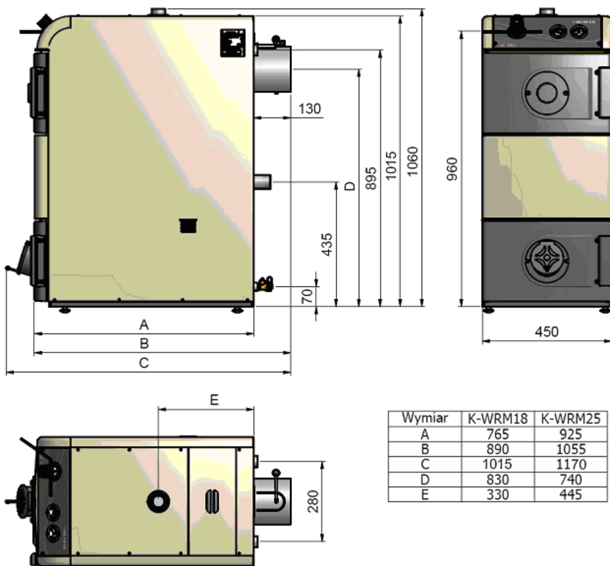
Рисунок 2. Размеры котла.
